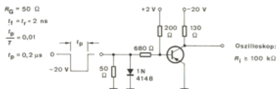
Meßschaltung für: t_d, t_r, t_{on}, t_s, t_f, t_{off}
