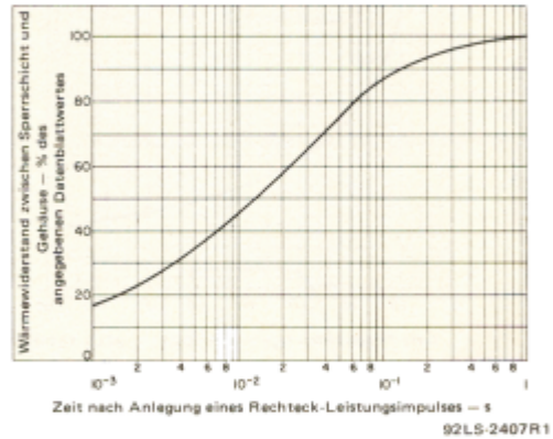
Bild 15 – Impulswärmewiderstand (Sperrschicht/Gehäuse) in Abhängigkeit von der Zeit
