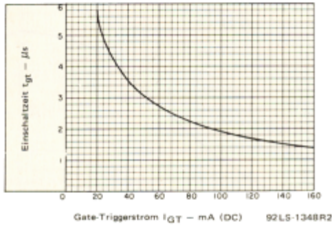
Bild 9 – Typische Einschaltkennlinie
