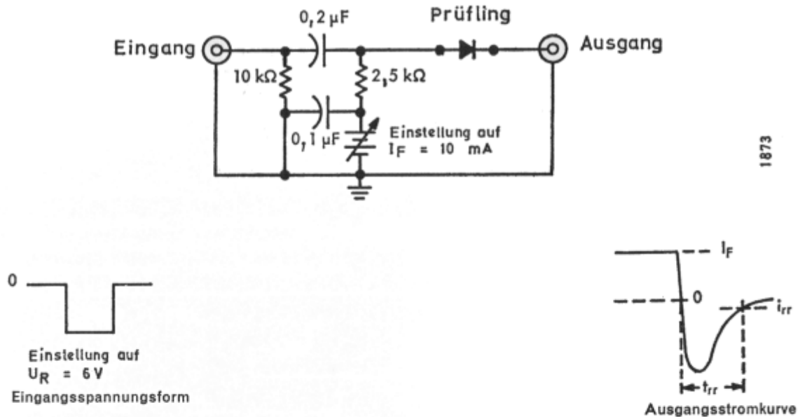
Bild 1 – Sperrverzögerungszeit
